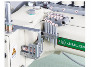
陶瓷过线结构 过线更顺畅，线迹更美观。
