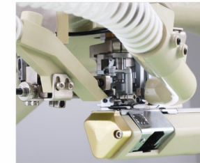
改进式断线刀具，安全不打手
